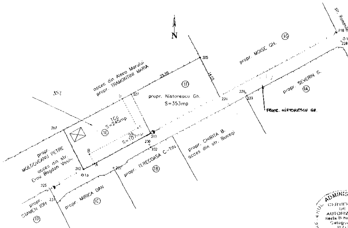
PLAN DE AMPLASAMENT SI DELIMITARE AL CORPULUI DE PROPRIETATE SCARA 1:500
